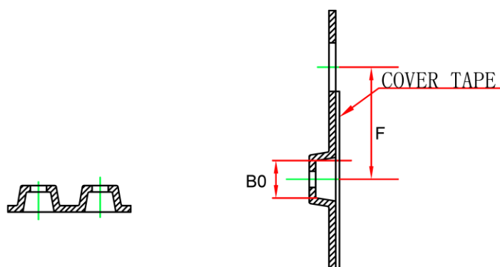
A - A
