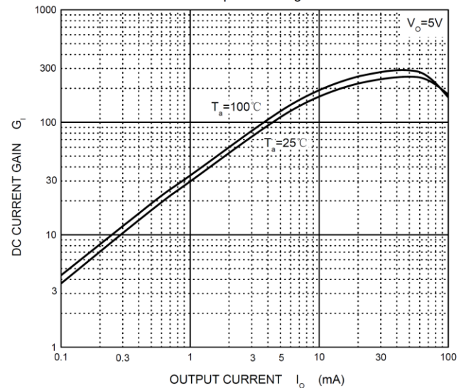
G_I — I_O
