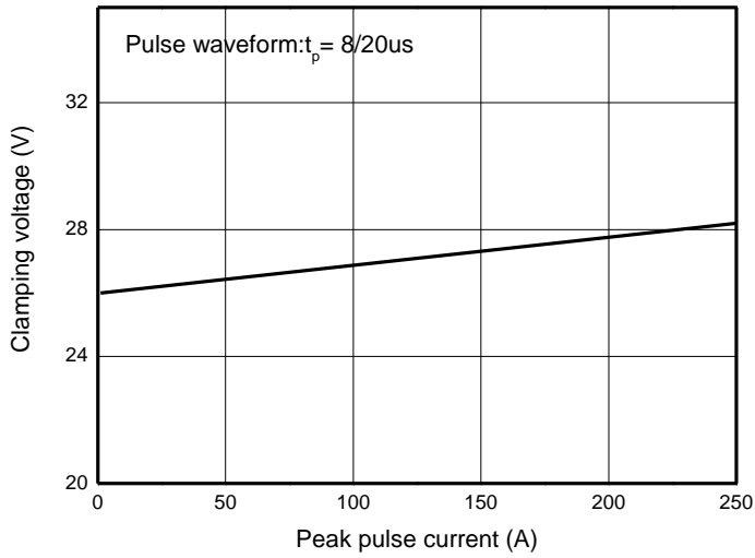
V_C vs. I_{PP}
